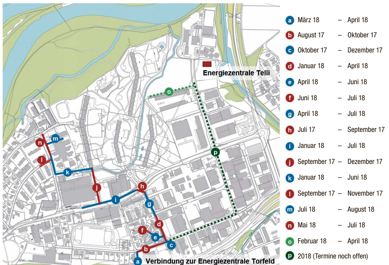
Abb. 3: Leitungsbau-Etappen vom Wärme- und Kälteverbund Telli
