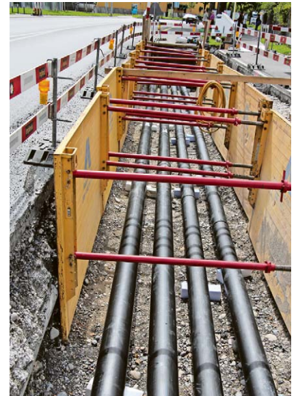
Strassenbaumassnahmen zum sicheren Verlegen der Leitungen
